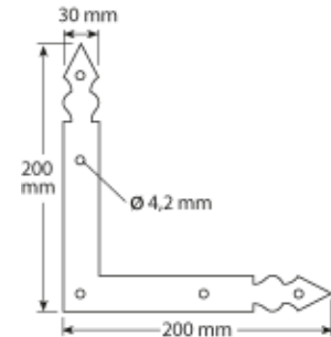
Eckwinkel
