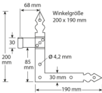
Winkelband gerade
