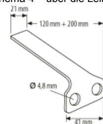
Riegelanschlag zu Ladenriegel (Schema 4 – über die Leibung)
