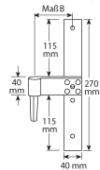
Winkelmitteband (Mitte Türflügel)
