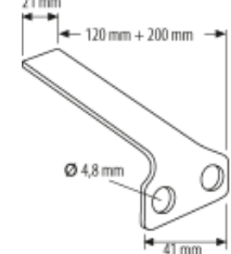
Riegelanschlag zu Ladenriegel (Schema 4 - über die Leibung)
