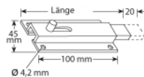
Standard-Ladenriegel (Länge 120+220 mm)
