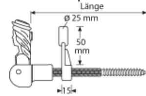
Kreuzband horizontal verstellbar (alternativ)
