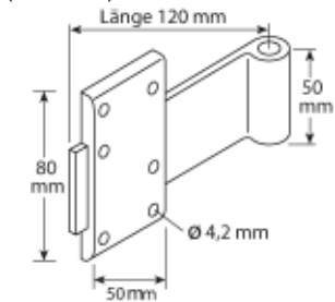
Kreuzband horizontal verstellbar (alternativ)
