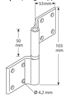
Standard-Ladenscharnier gekröpft (bei gekuppelten Läden)
