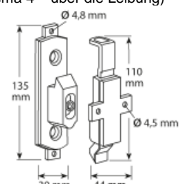
Ladenhalter für gekuppelte Türläden (Schema 4 - über die Leibung)
