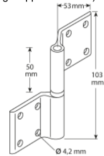
Ladenscharnier gekröpft (bei gekoppelten Läden)
