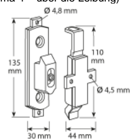
Ladenhalter für gekoppelte Türläden (Schema 4 – über die Leibung)
