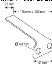
Riegelanschlag zu Ladenriegel (Schema 4 – über die Leibung)
